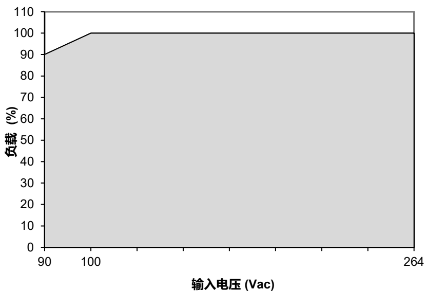
图. 2 AC 输入电压功率降额 < 100 Vac 功率降额 1% / Vac
