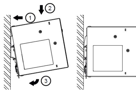
图. 3.1 安装
