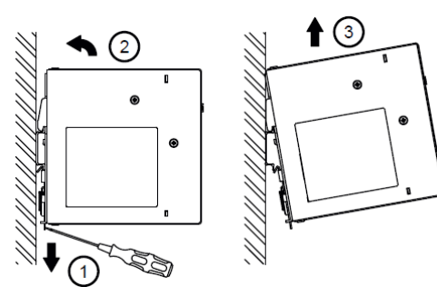
图. 3.2 拆卸
