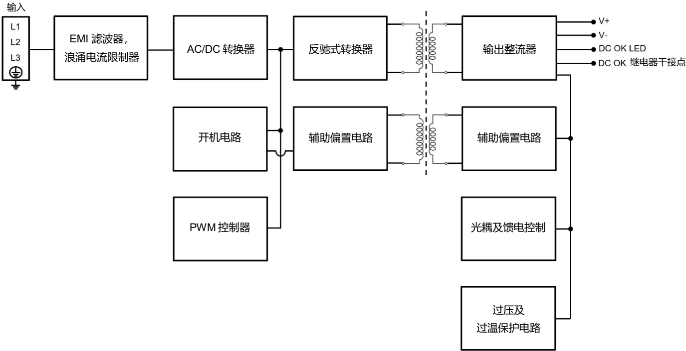
方块图
