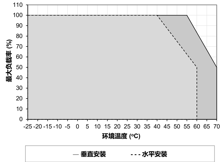
输出负载降额对应环境温度
